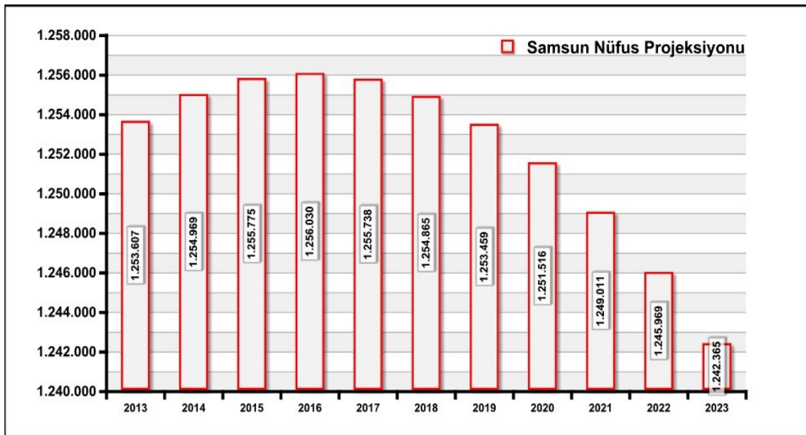
Grafik2: Samsun Nüfus Projeksiyonları
