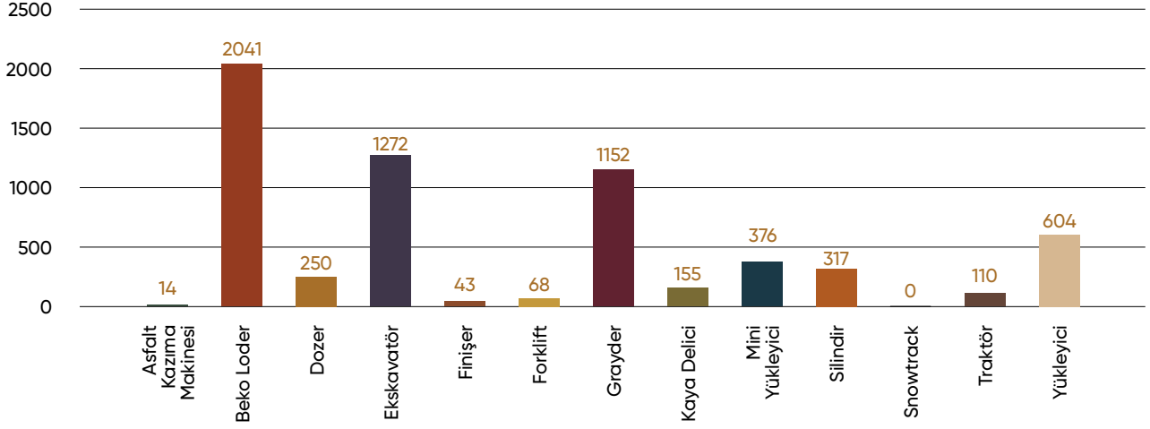
ARIZALARIN MAKİNE SINIFLARINA GÖRE DAĞILIMI
